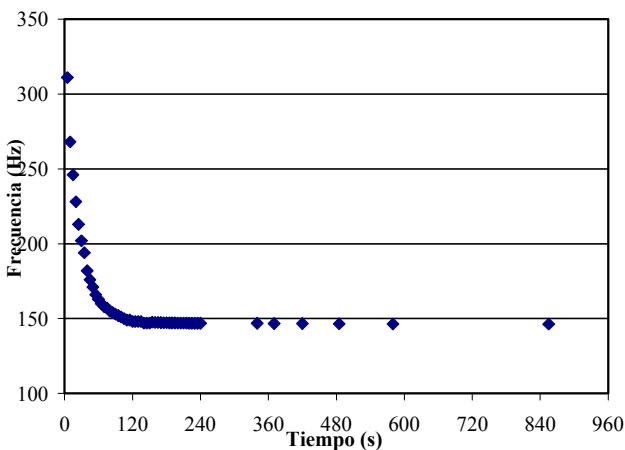
Figura 7: Tiempo de estabilización de la sonda en C.C.
