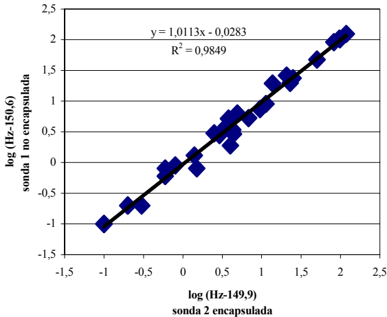
Figura 6: Comparación de una Sonda encapsulada con una no encapsulada
